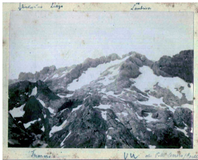
En 1872, la extensión del hielo glacial y de los neveros del Jou Tras Llambrión probablemente era semejante a la se ve en esta fotografía, tomada por el conde de Saint Saud veinte años más tarde. (Notas manuscritas de Saint-Saud y G. Schulze).
